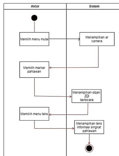
Gambar 5. Activity Diagram Memulai Aplikasi
