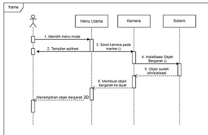
Gambar 8. Sequence Diagram Cara Menjalankan Program
